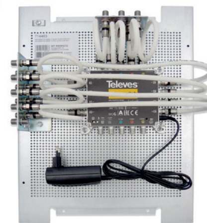
PRZYKŁADOWA INSTALACJA MULTISWITCHA
